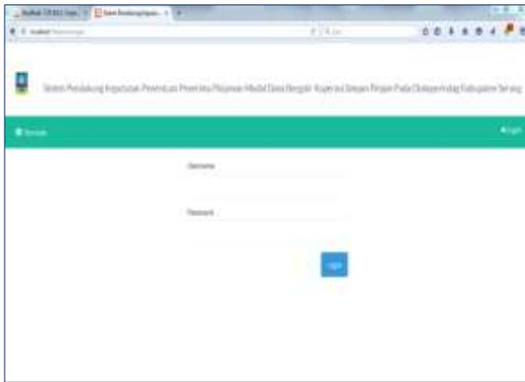
Gambar 4.1 Login
