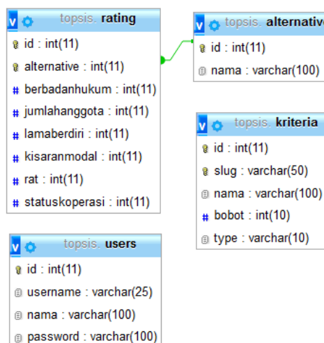
Gambar 3.2 Rancangan Database
