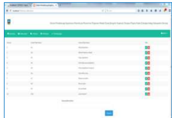
Gambar 4.4 Alternatif
