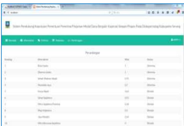
Gambar 4.3 Beranda Admin
