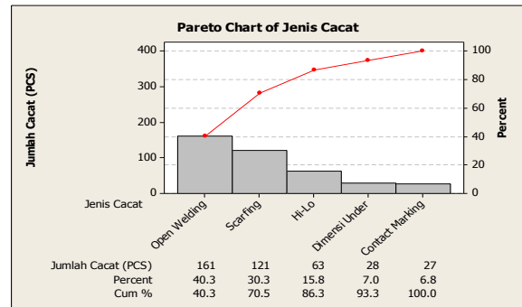
Gambar 3. Diagram Pareto Kecacatan Pipa API 5L
