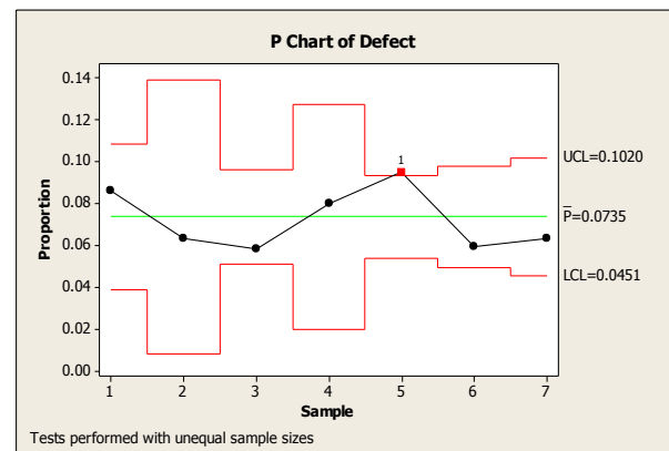
Gambar 2. Grafik Peta Kendali
