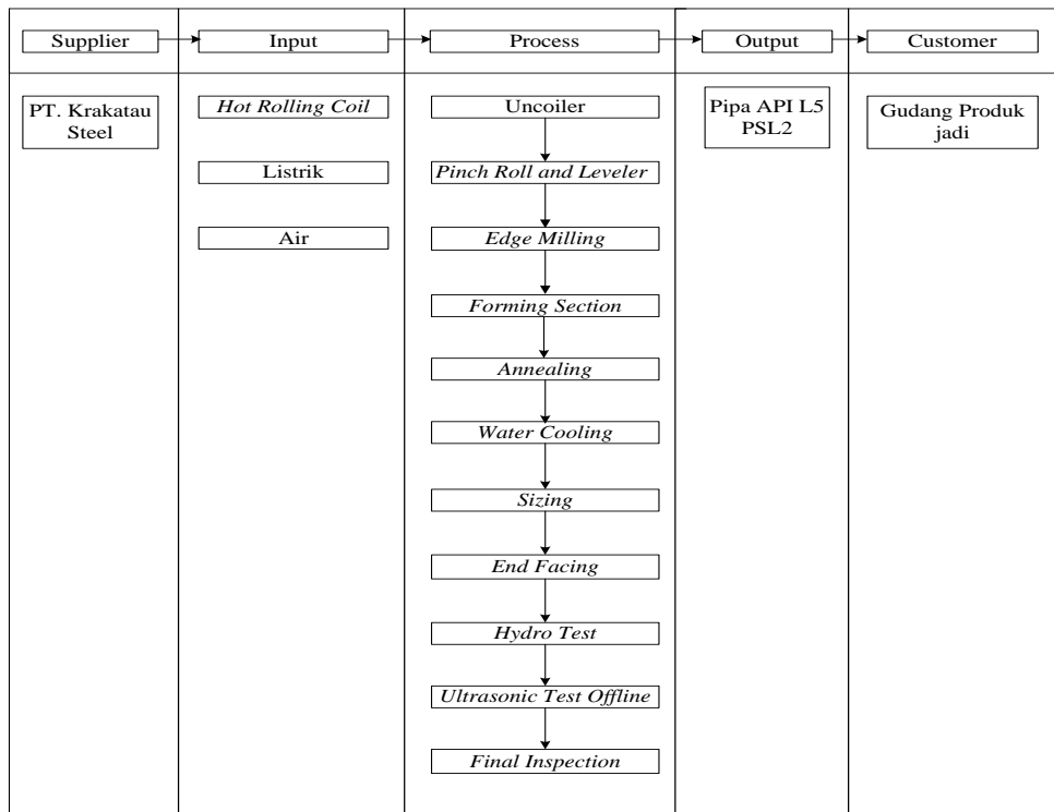
Gambar 4.3 Diagram SIPOC proses produksi pipa API 5L PSL2
