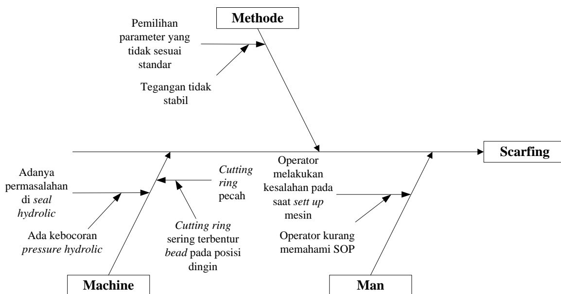
Gambar 5. Diagram sebab akibat kecacatan Scarfing
